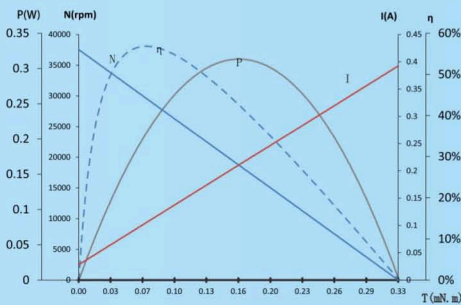
Model: 0610RN55-8-30A1-3.5
