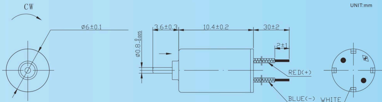
Model: 0610RN55-8-30A1-3.5
