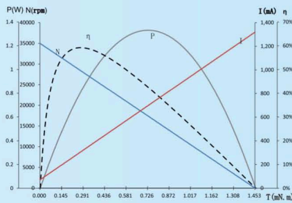
Model : 1013RN01-10L97-4.5
