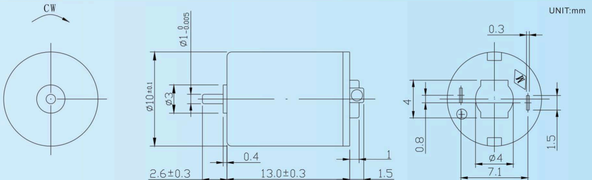
Model : 1013RN01-10L97-4.5
